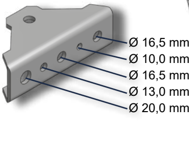
Lochbild Endgelenk
